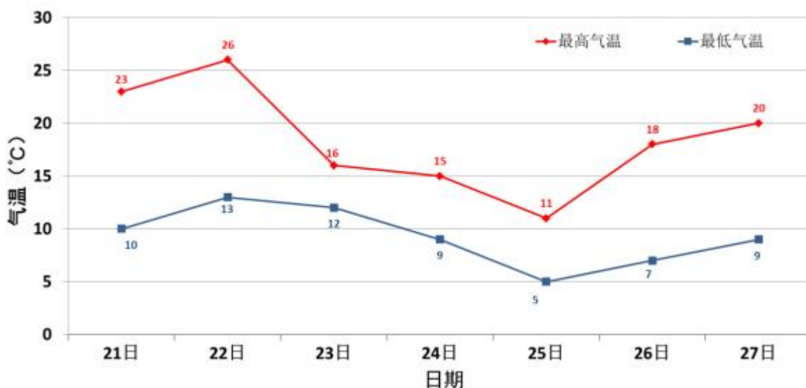
图1 2024年3月21~27日唐河站最高气温（红线）、最低气温（蓝线）预报图（℃）
